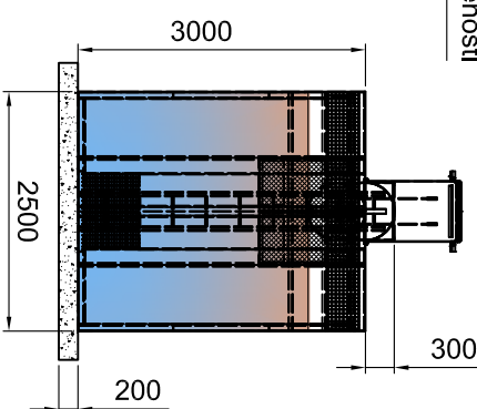
Regulacija kliznih grla vijcima M12x25
